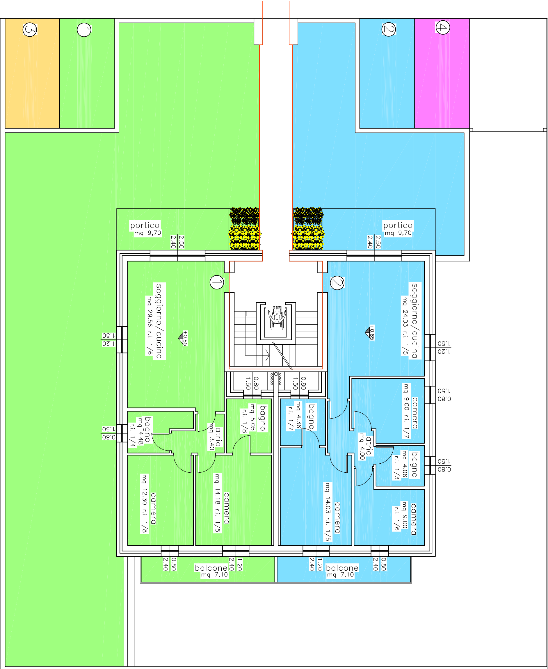
PIANTA PIANTERRENO
